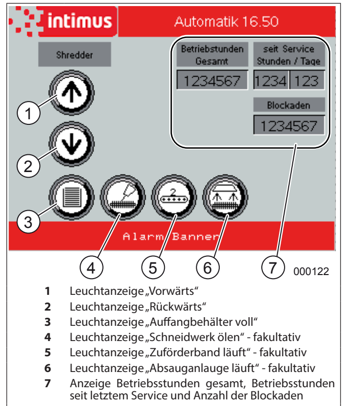
Abb. 7 Bildschirm Automatikbetrieb
