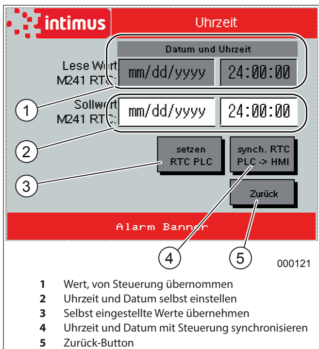
Abb. 6 Bildschirm Datum-Uhrzeit
